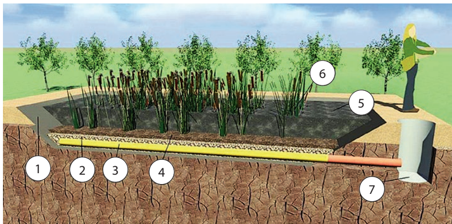
Schéma trstinového kalového poľa KČOV (Vysvetlivky: 1 – izolačná fólia, 2 – drenážna vrstva, 3 – odvodňovacie potrubie, 4 – pieskový substrát, 5 – odvodňovaný kal, 6 – mokračové rastliny, 7 – zberná šachta na vodu (na čerpanie alebo kontrolu, odtok do čistiarene). Autor: Michal Kriška Dunajský
